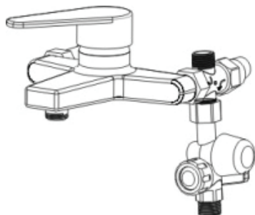
Рисунок 18. Схематическое отображение после установки обратного клапана с сетчатым фильтром
